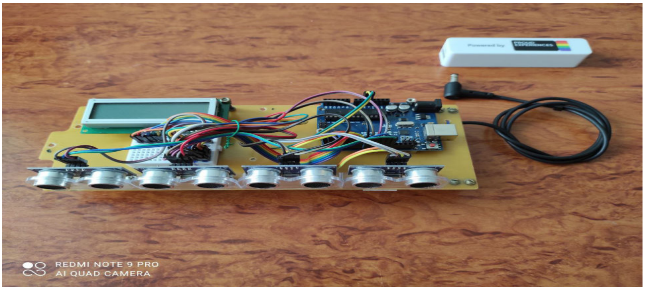
Рис. 2. Технічна реалізація ІВС для визначення профілю будівельних конструкцій
