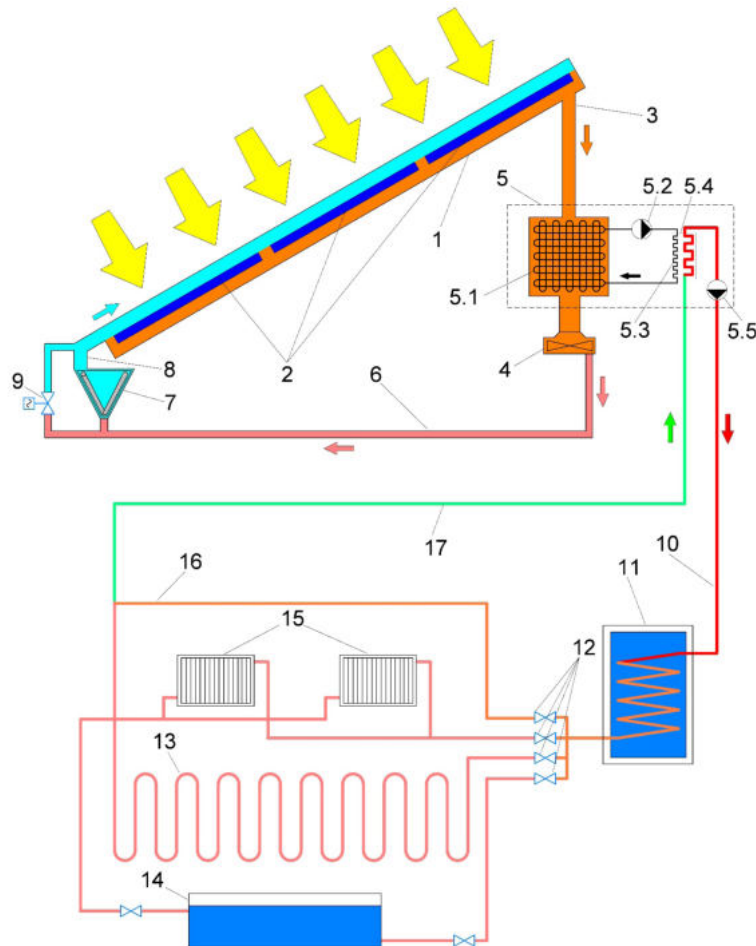
Рис. 1. Схема ГЕУ з охолодженням сонячних модулів
