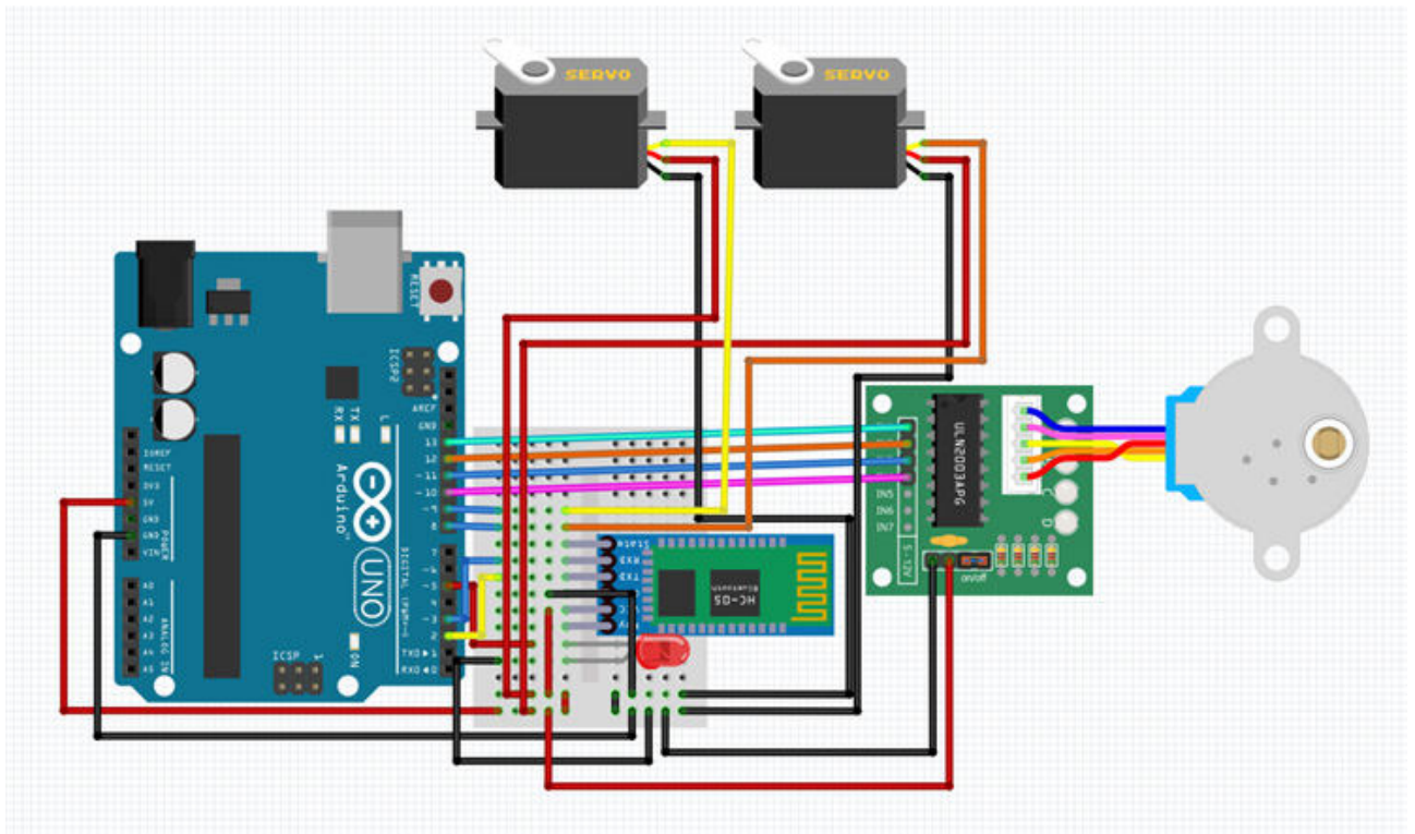
Рис. 1. Схема під'єднань елементів системи керування камерою
