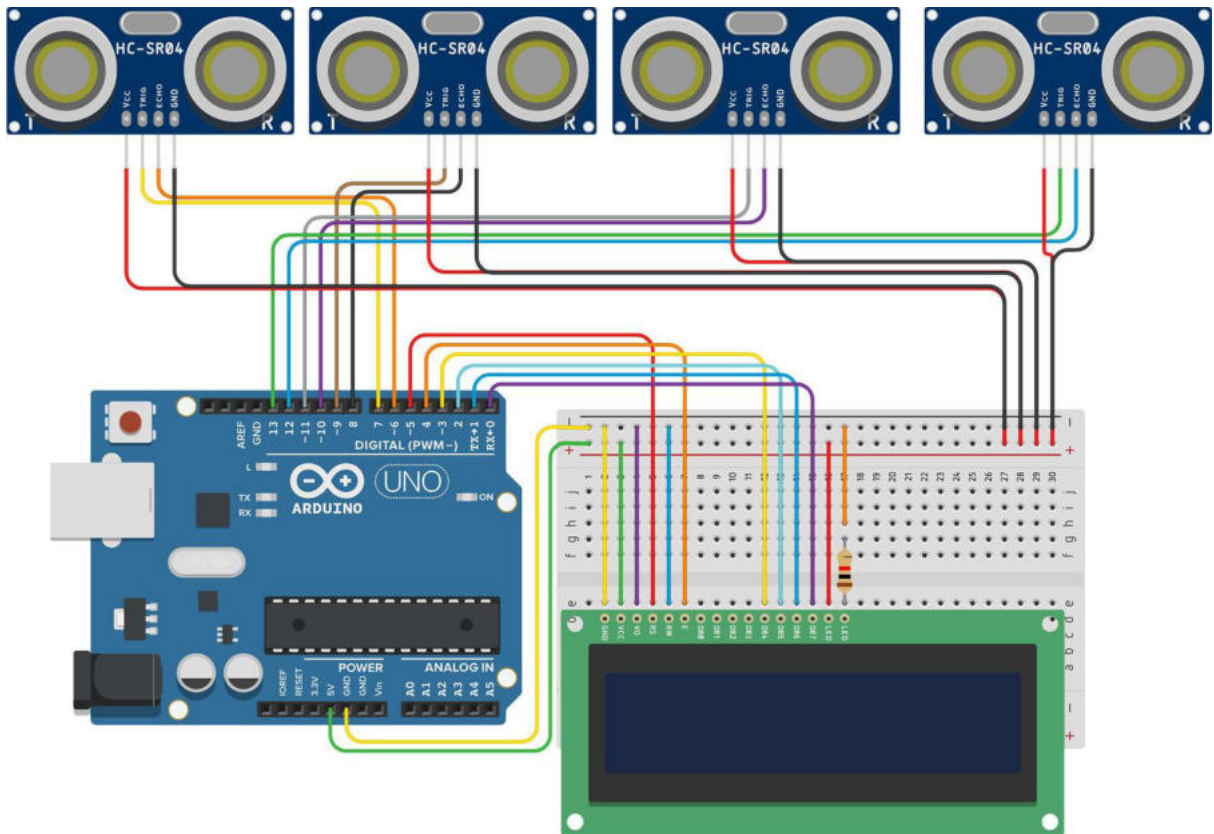
Рис. 1. ІВС для визначення профілю будівельних конструкцій
