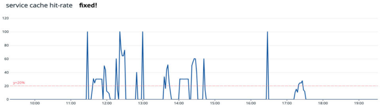
Рис.3 Графік оберненого моніторингу cache hit rate
