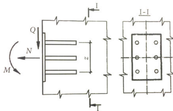
Рис. 3. Схема зусиль, які діють на закладну деталь.
