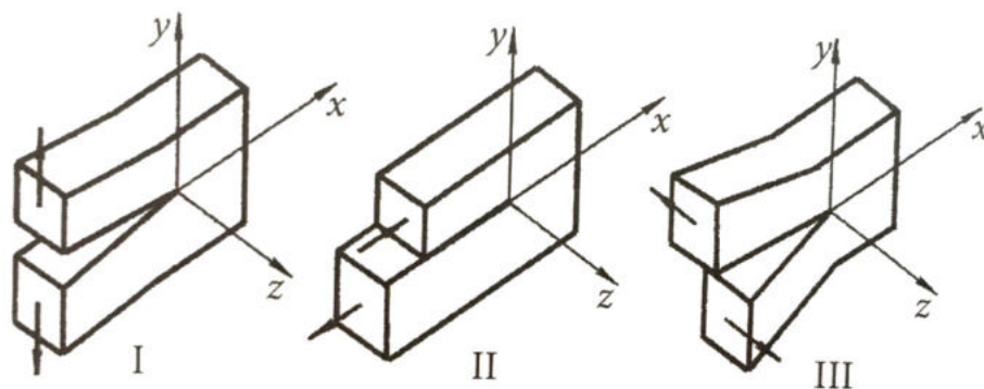
Рис. 4. Різновиди переміщення берегів тріщин і відповідно руйнувань:
