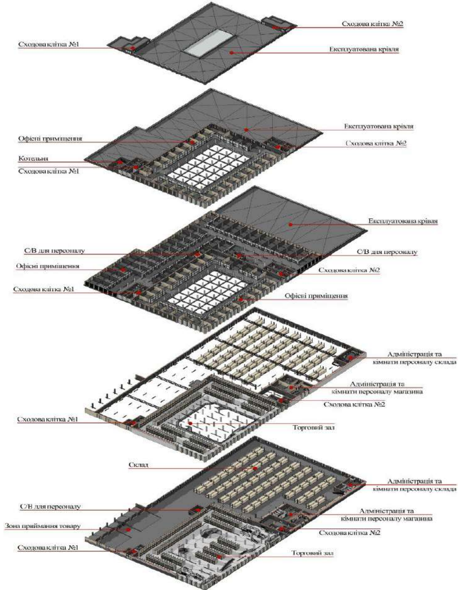
Рис. 3. Вибух-схема проектного будівельного хабу.
