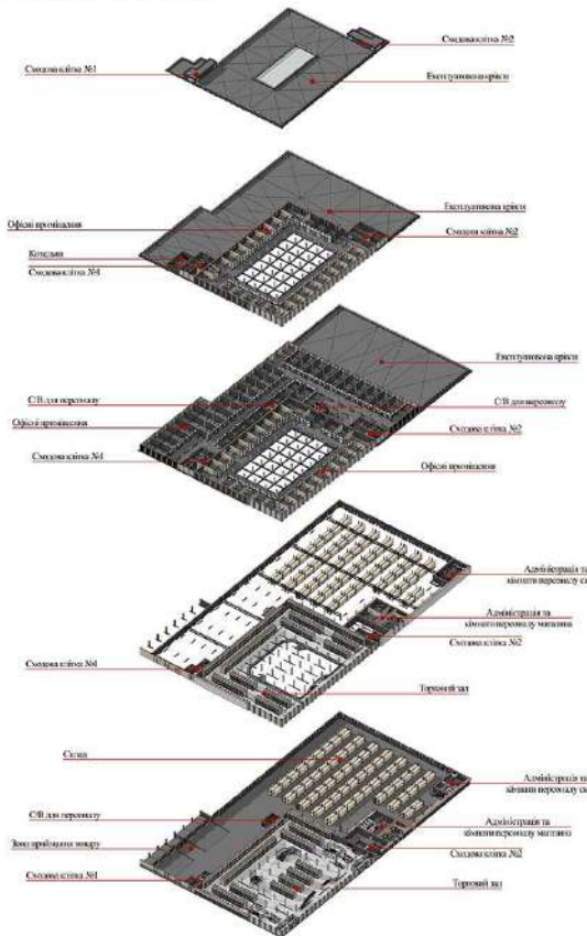
Схема планування будівельного хабу
