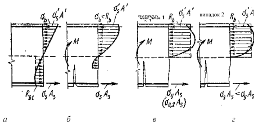
Рис.1 – Три стадії напруженого стану залізобетонних елементів при згині: а – I стадія – пружна; б – II стадія – робота з тріщинами; в – III стадія – руйнування по арматурі; г – III стадія – руйнування по бетону
