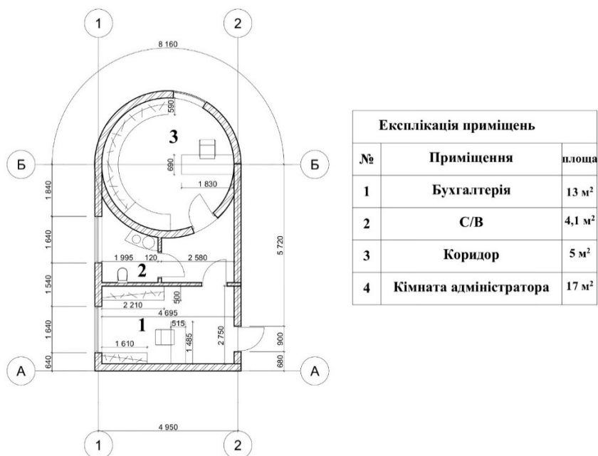
Рис. 3. Планування закинутого приміщення водонапірної бапти.
