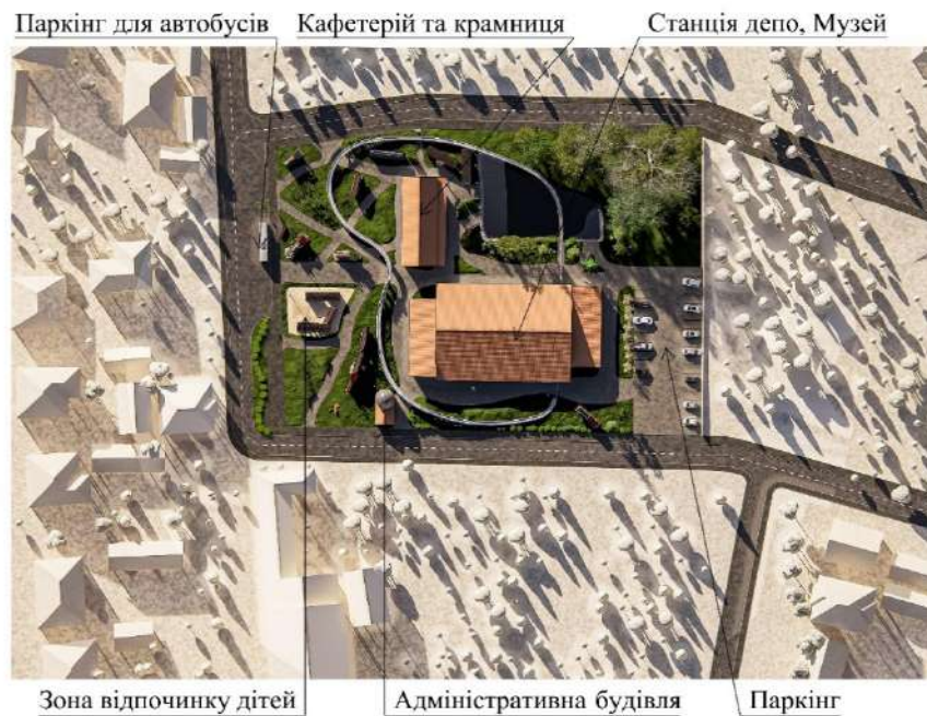
Рис. 2. Схема функціональної організації території вузькоколієного депо.
