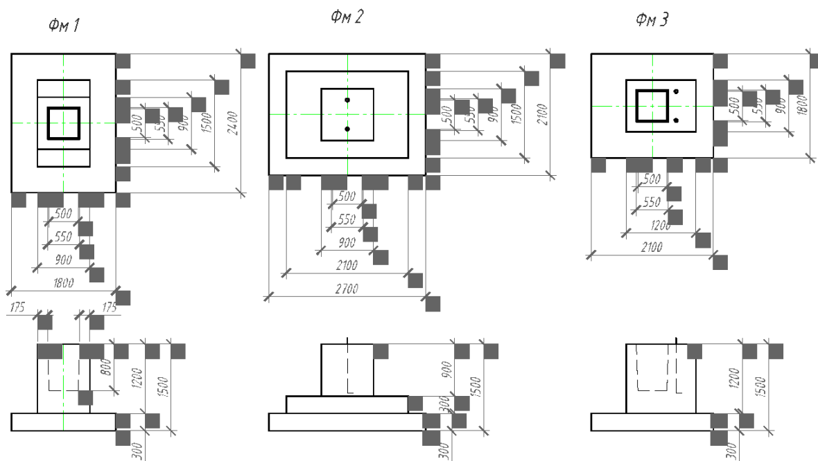
Малюнок 1.11 - Залізобетонні монолітні фундаменти
